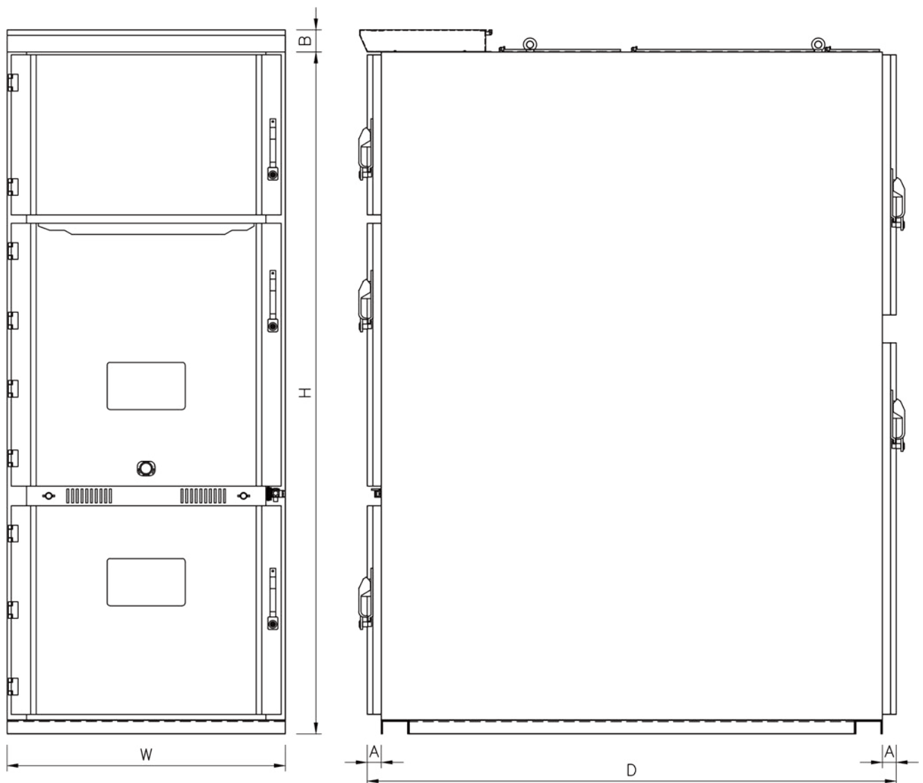
尺寸 Dimensions 單位Unit : mm
