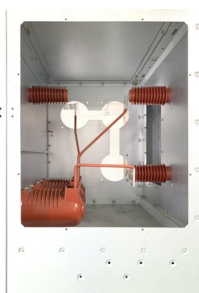
匯流排分隔室
