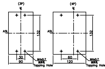
固定孔位 Drilling Plan
