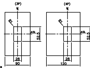
鑿面孔面 Panel Cutout
