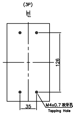
固定孔位 Drilling Plan
