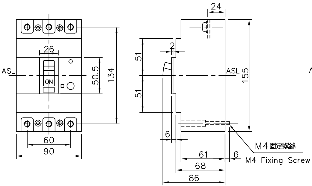
TLB-125E 外形尺寸圖
