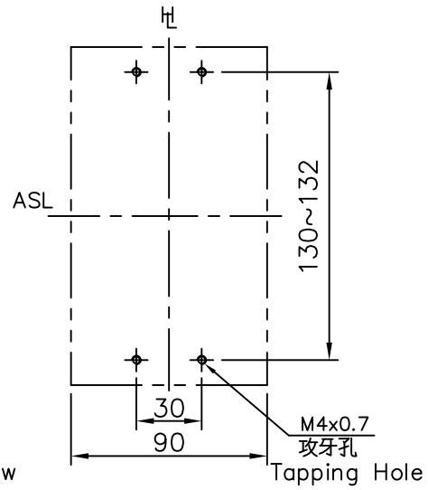
固定孔位 Drilling Plan
