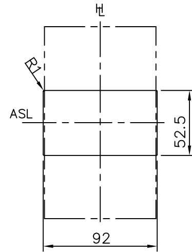
盤面孔位 Panel Cutout
