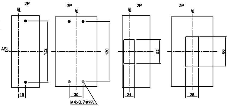
固定孔位
