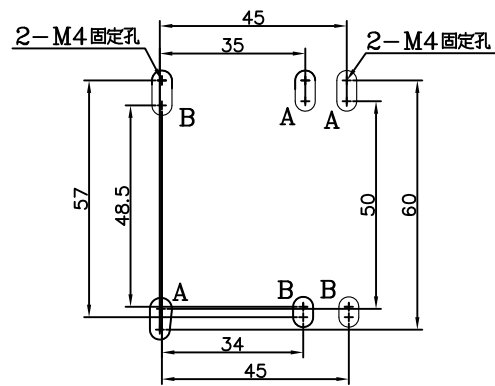
固定尺寸
