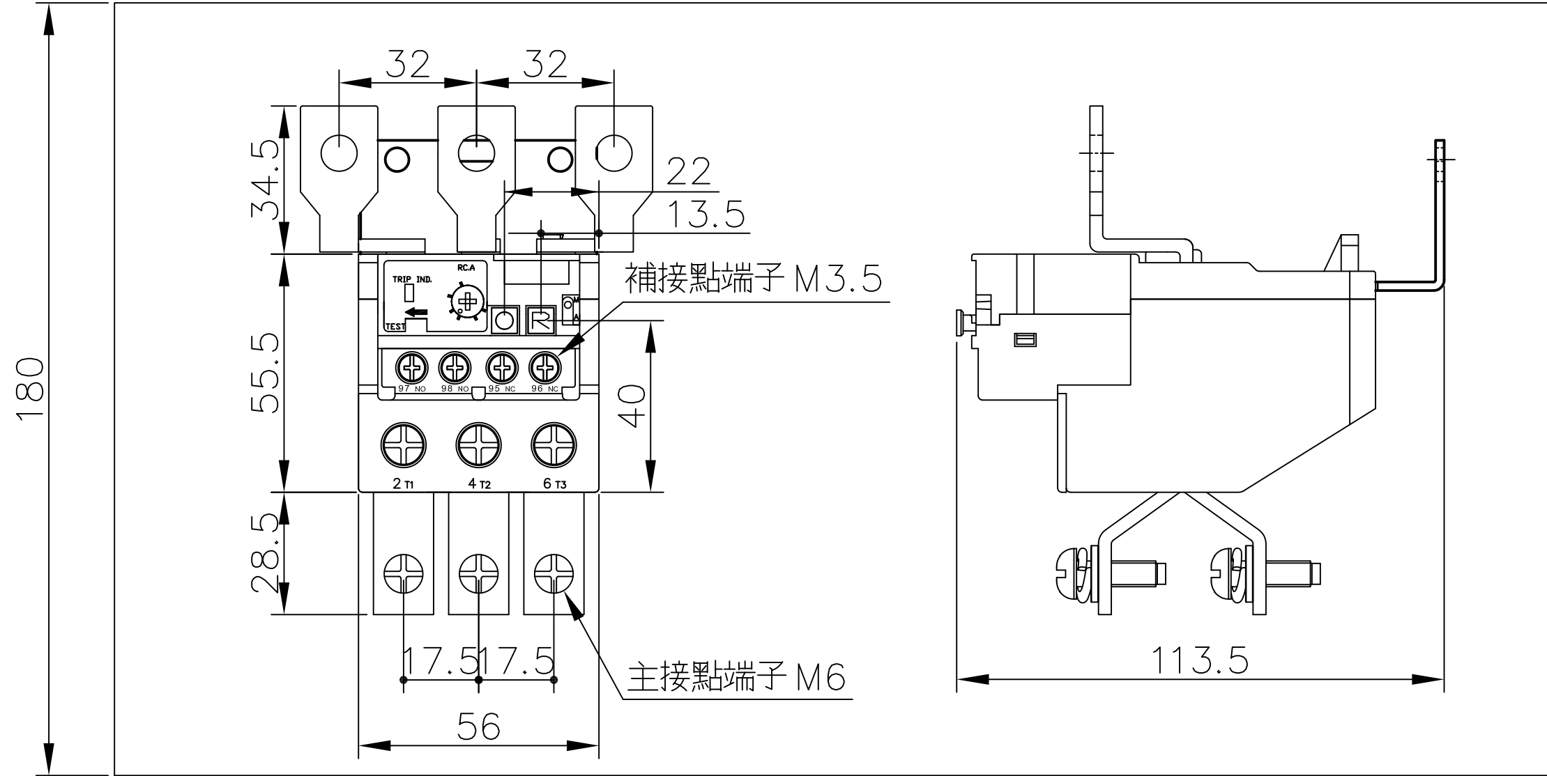
RHU-80/□ 5 外形圖尺寸
