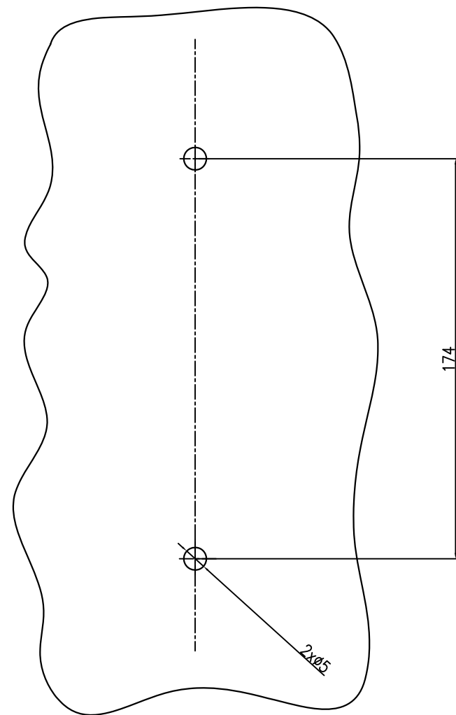
安裝板開孔圖
