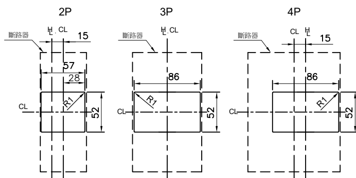
固定孔位 Drilling Plan
