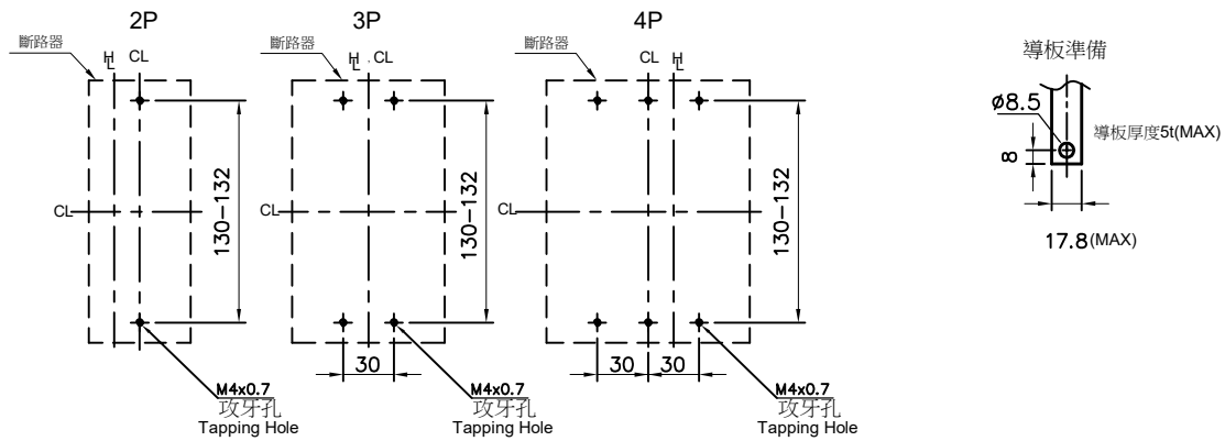
固定孔位 Drilling Plan
