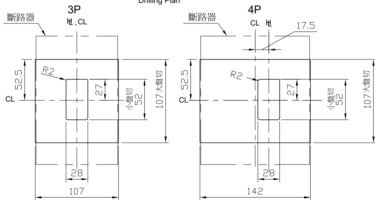
盤面孔位 Panel Cutout
