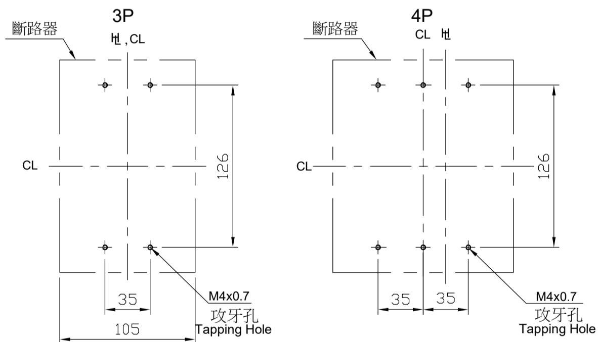
固定孔位 Drilling Plan
