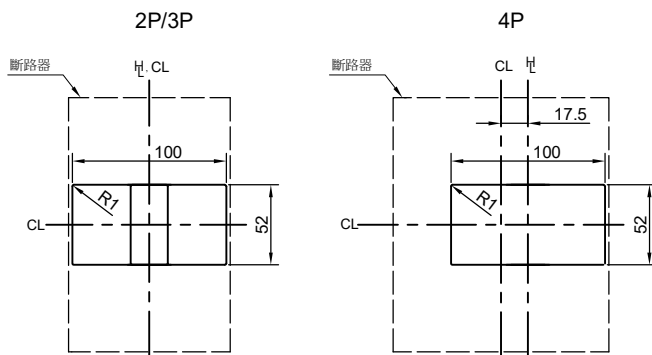
盤面孔位 Panel Cutout
