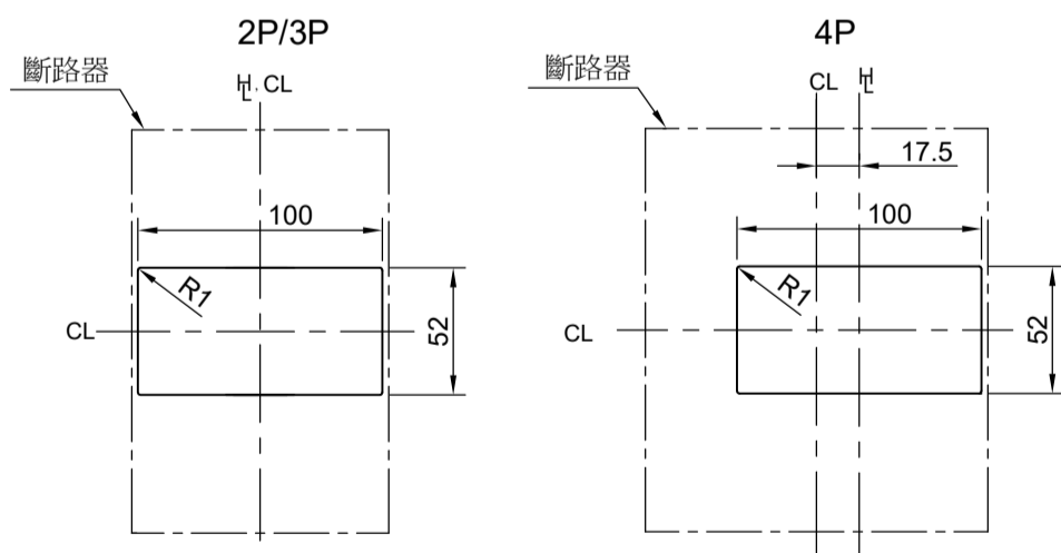
盤面孔位 Panel Cutout
