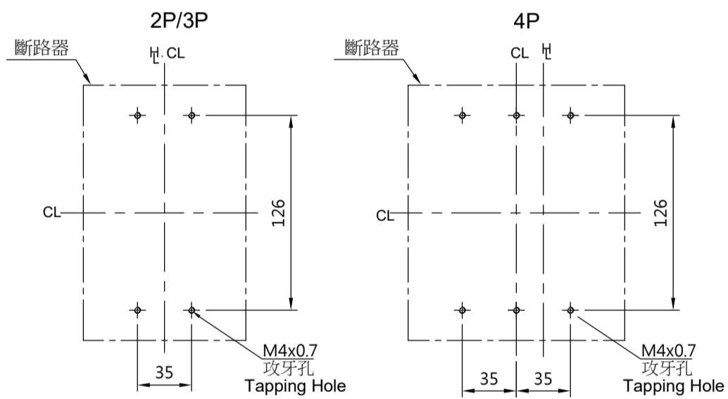
固定孔位 Drilling Plan
