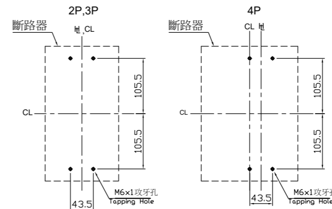
固定孔位 Drilling Plan
