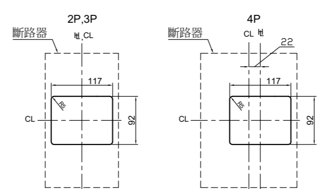
盤面孔位 Panel Cutout
