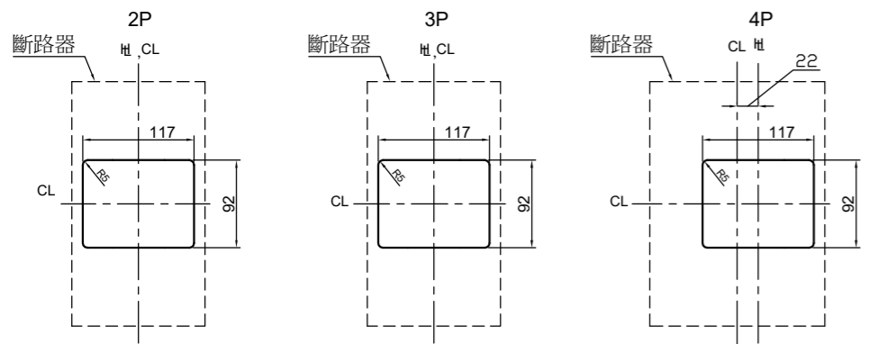
盤面孔位 Panel Cutout
