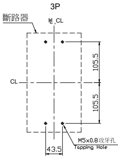
固定孔位 Drilling Plan
