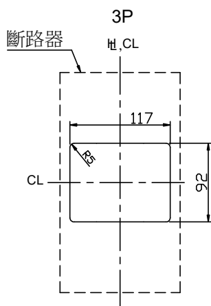
固定孔位 Drilling Plan
