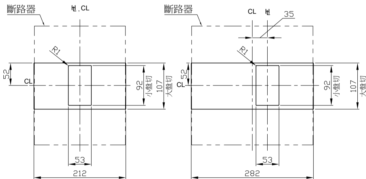
盤面孔位 Panel Cutout
