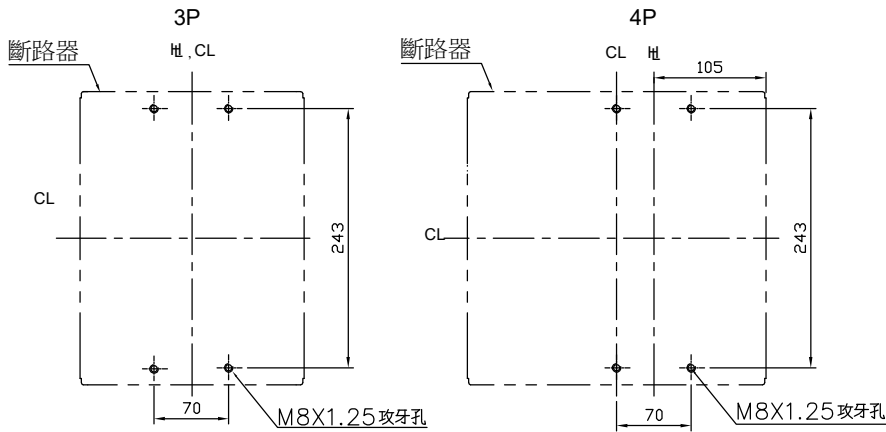
固定孔位 Drilling Plan
