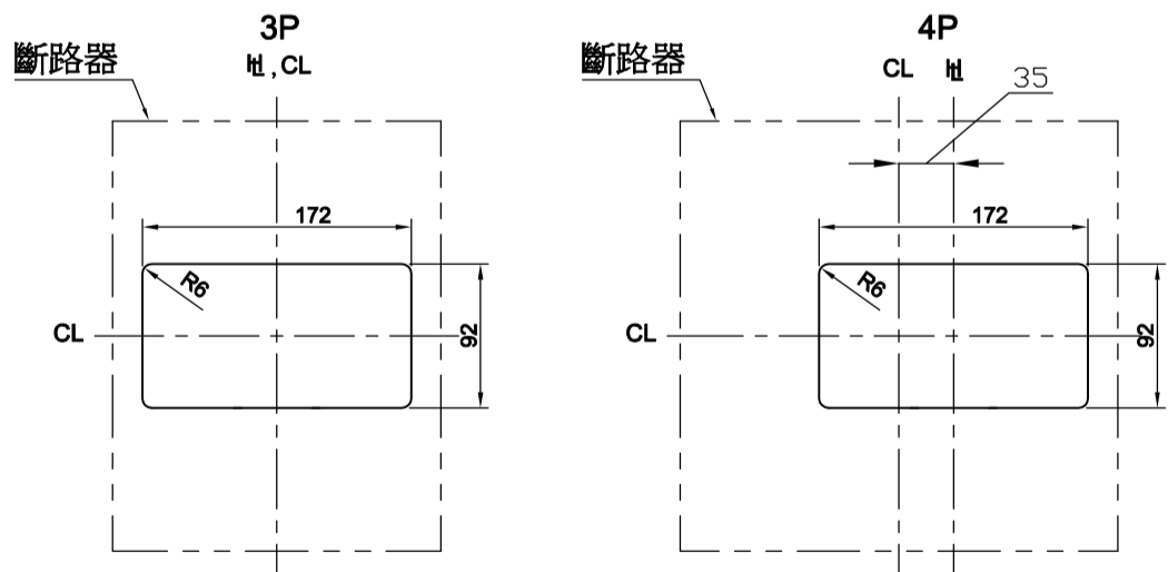
固定孔位 Drilling Plan
