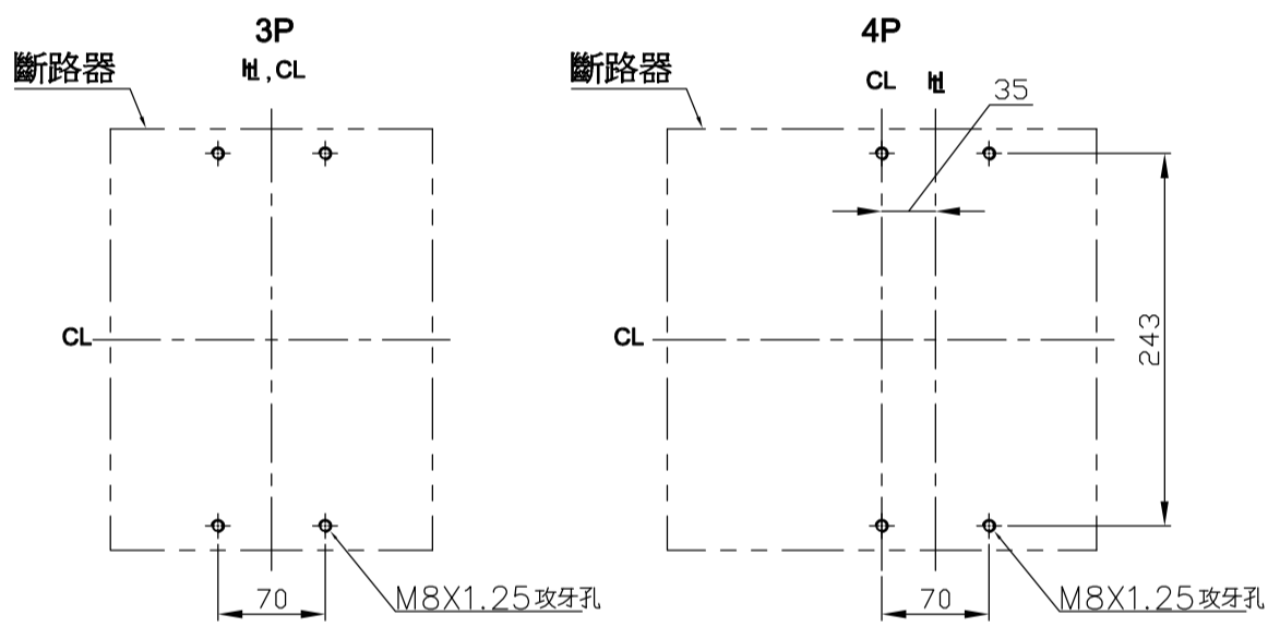
固定孔位 Drilling Plan
