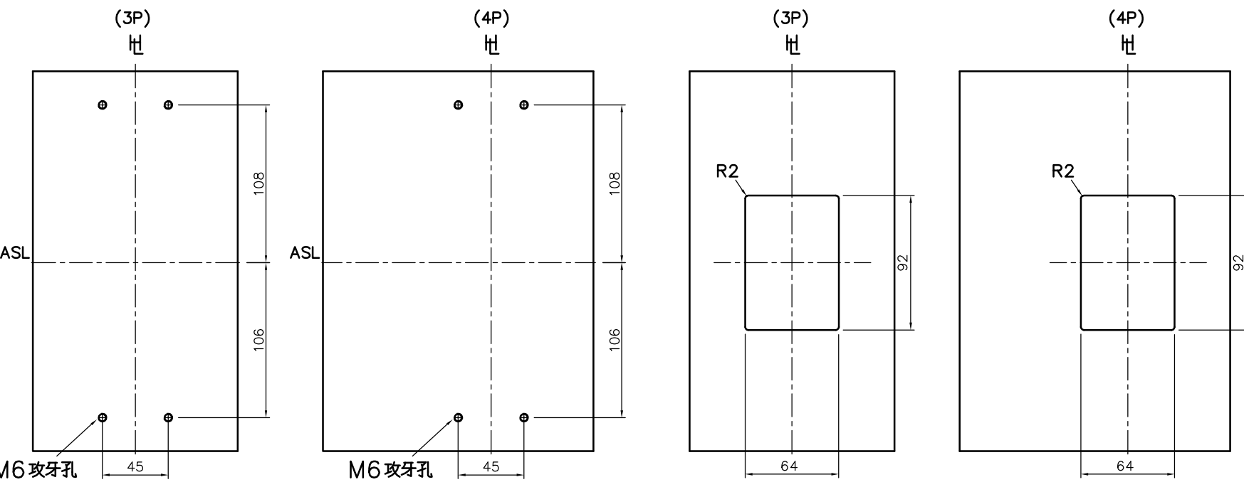
固定孔位 Drilling Plan
