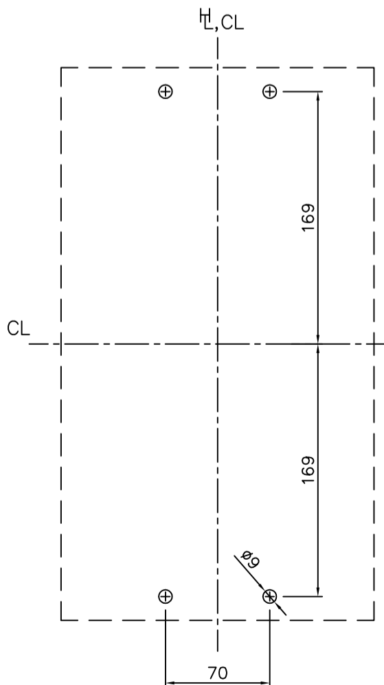
固定孔位 Drilling Plan
