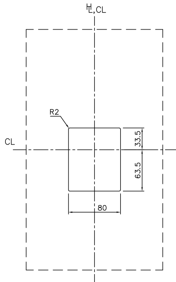
盤面孔位 Panel Cutout
