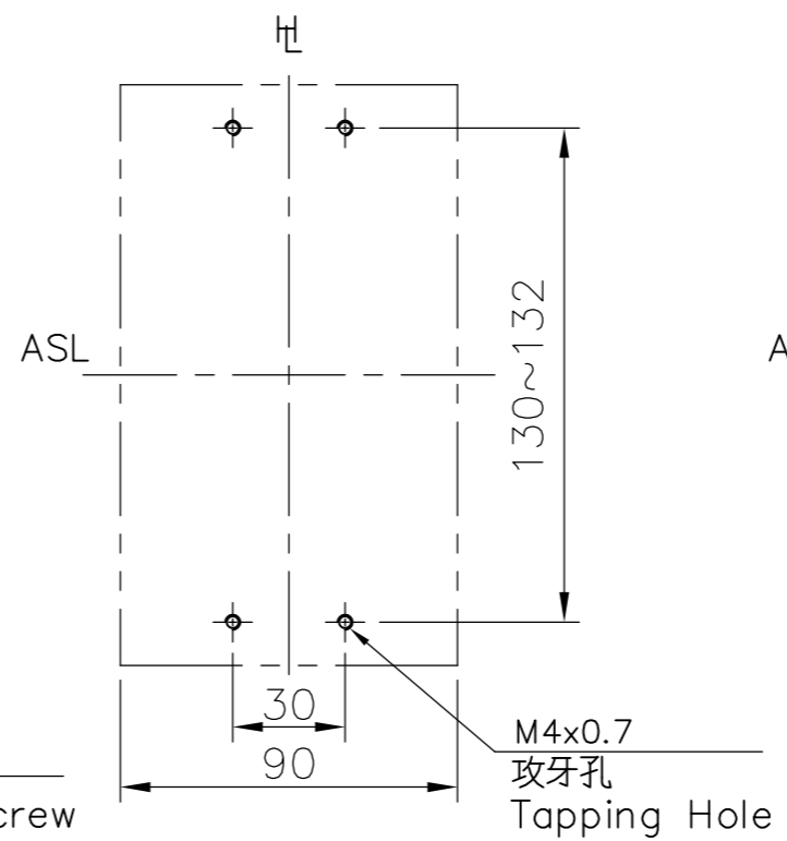
固定孔位 Drilling Plan
