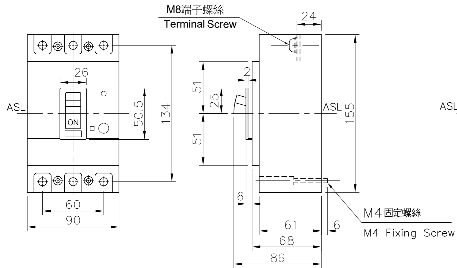
TLB-125E 外形尺寸圖
