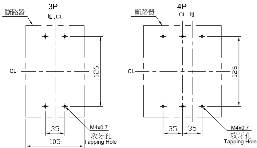
固定孔位 Drilling Plan
