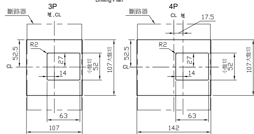
盤面孔位 Panel Cutout
