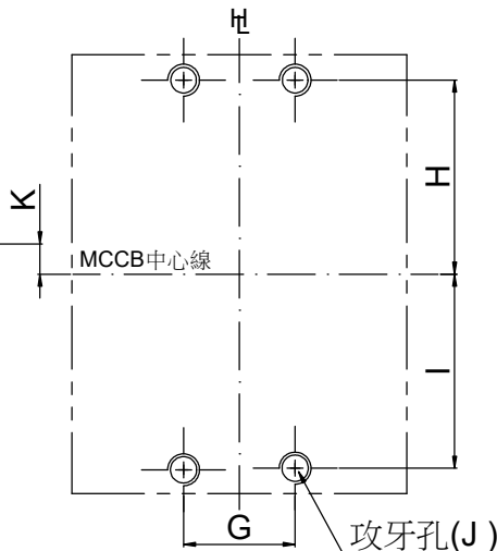
MCCB固定孔
