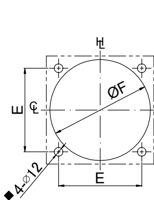
盤面孔位
