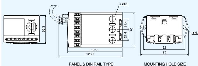
EOCR-FDM2-HZ(過孔式)
