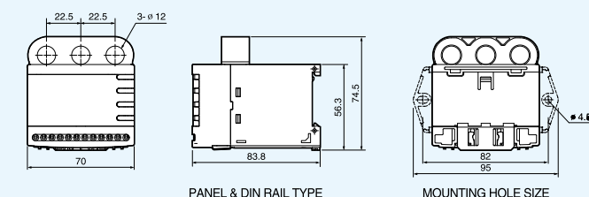
(穿線式)
