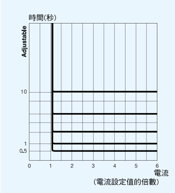
EOCR-SSD的定時限特性
