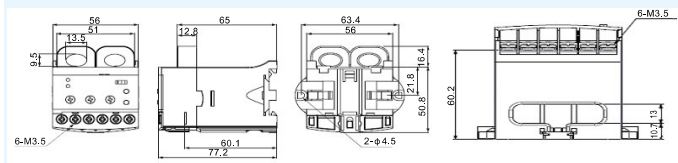
EOCR-SS
