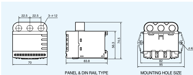
EOCR-i3DM-WZ / i3M420-WZ (穿線式)
