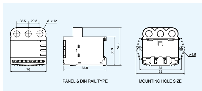
EOCR-3DM2-WZ(穿線式)
