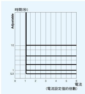
EOCR-SSD的定時限特性
