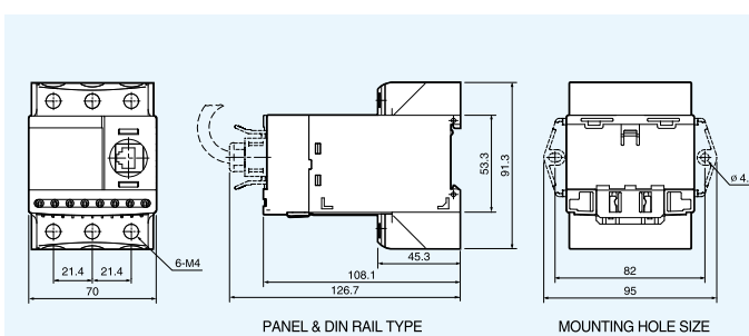
EOCR-FDM2-TZ(端子式)
