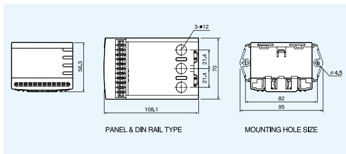
EOCR-i3DM-HZ / i3M420-HZ (過孔式)
