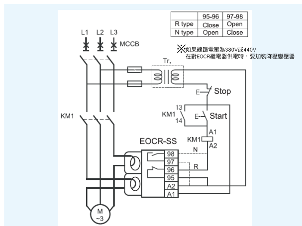
EOCR-SS
