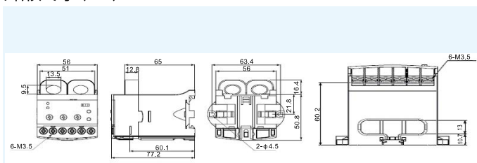
EOCR-SS
