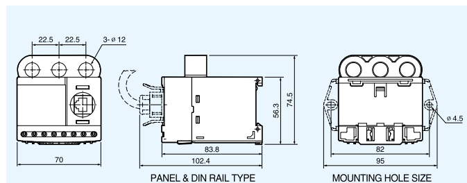
EOCR-FDM2-WZ(穿線式)
