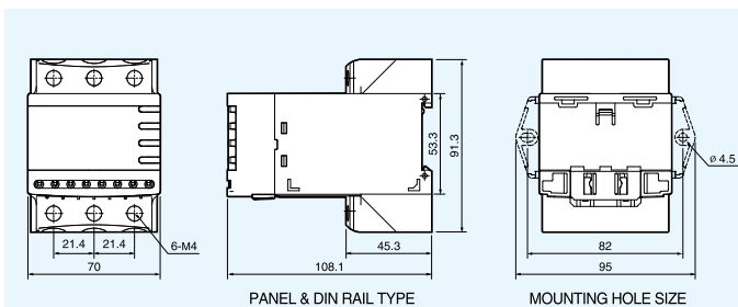
EOCR-3DM2-TZ(端子式)
