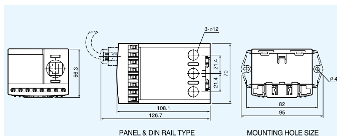
EOCR-FDM2-HZ(過孔式)
