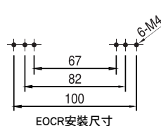
EOCR安裝尺寸
