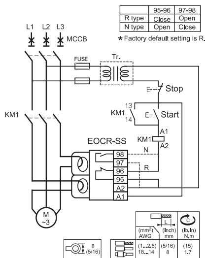
EOCR-SS 接線參考圖
