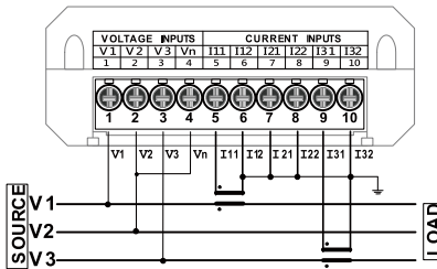
三相三線：無PT/2CT
