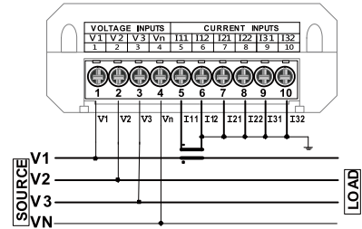
三相四線：無PT/1CT
