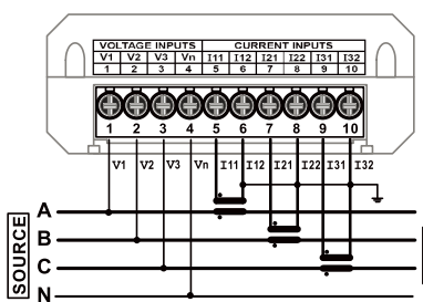
3P4W-電壓直入無PT/3CT[設定:3P4Y]
