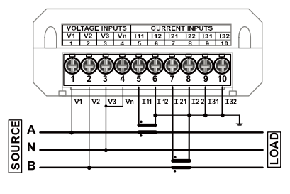
1P3W-無PT/2CT[設定:1P3Y]
