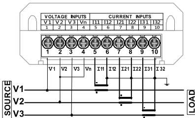
三相三線：無PT/3CT
