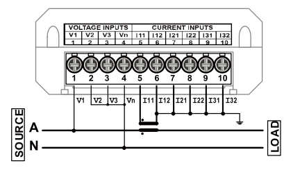
1P2W-無PT/1CT[設定:1P2Y]
