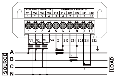
3P4W-3PT/3CT[設定:3P4Y]
