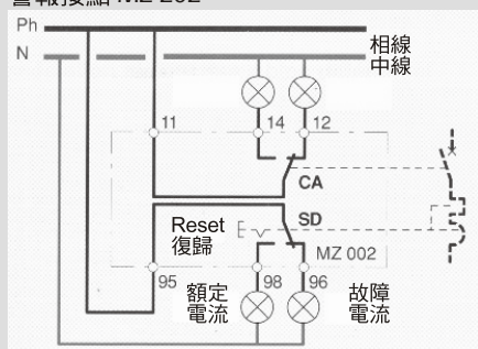
C A 輔助功能 S D 警報接點
