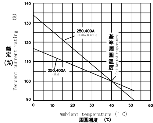
TG-400HJ 溫度補正曲線圖
