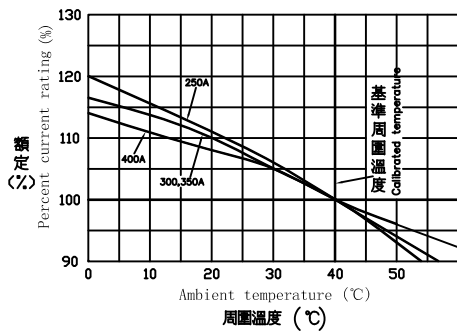
TG-400HB 溫度補正曲線圖
