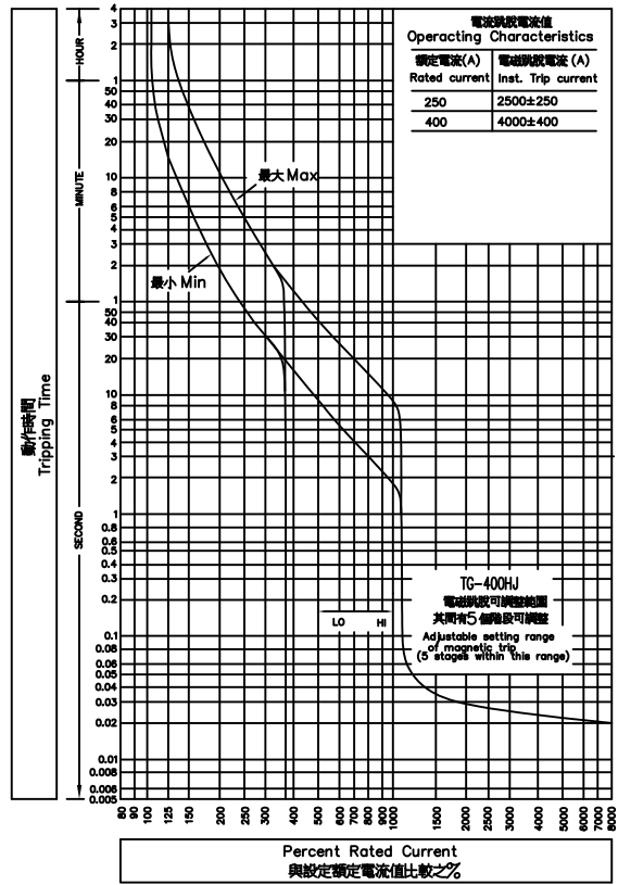
TG-400HJ 動作特性曲線圖
