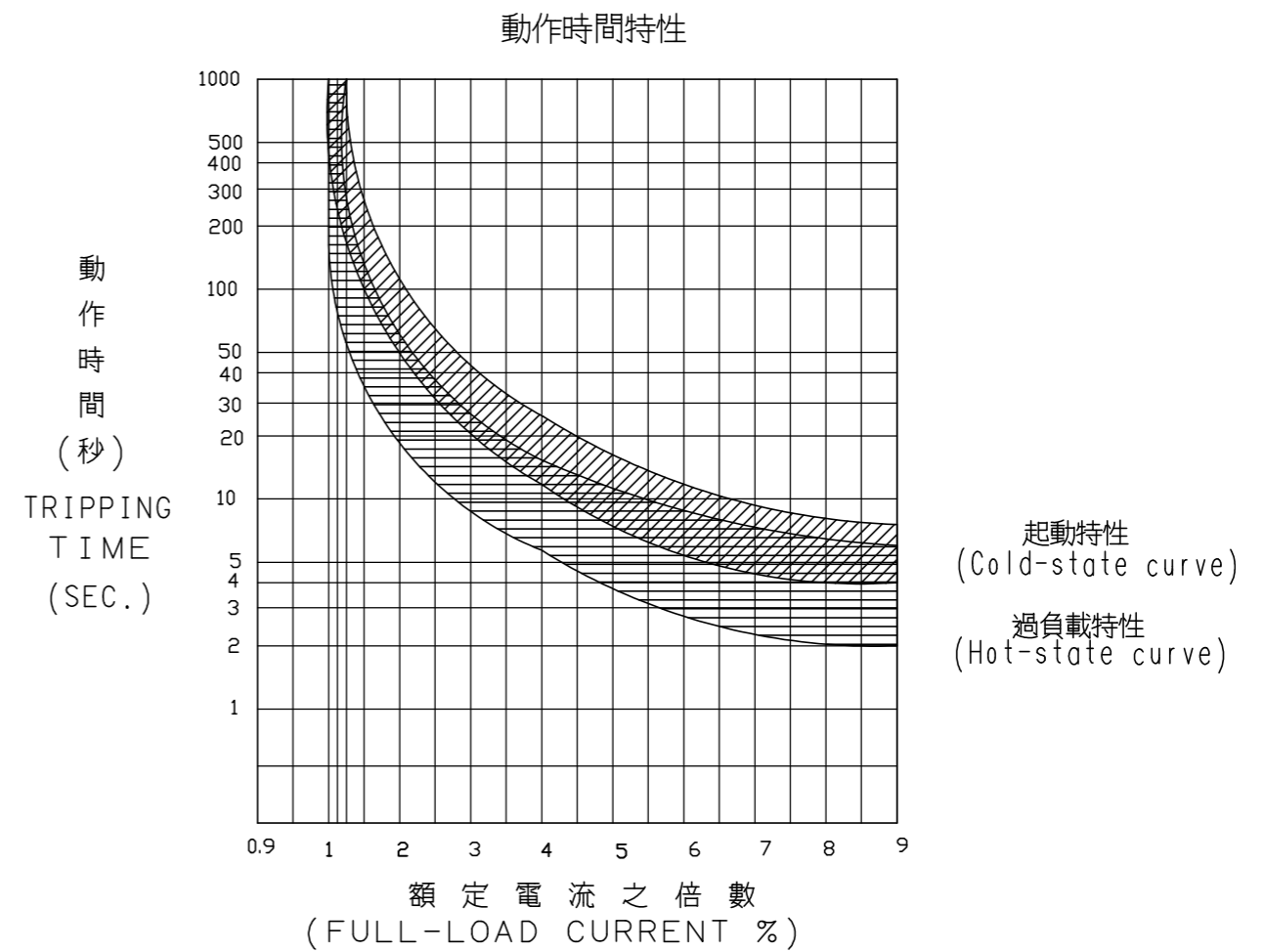
三相健全時之動作時間特性
