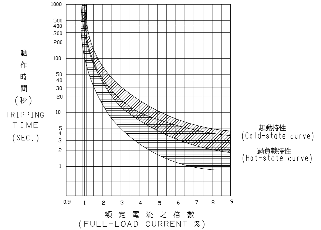
欠相時之動作時間特性
