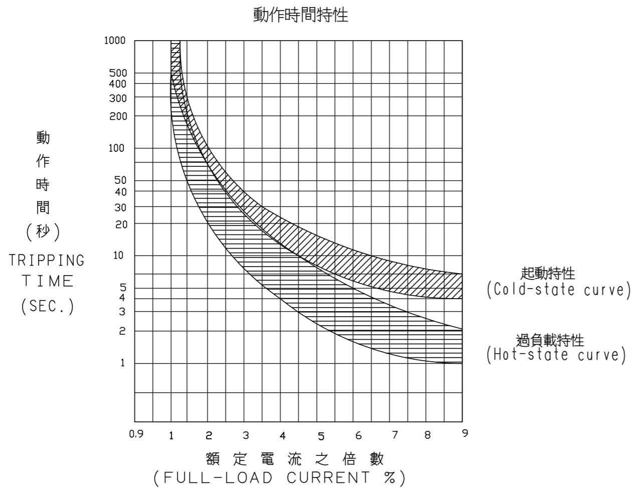
三相健全時之動作時間特性
